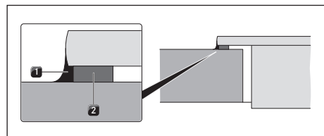
Abb. 10.24 Dichtungsband bei Aufsatzmontage
