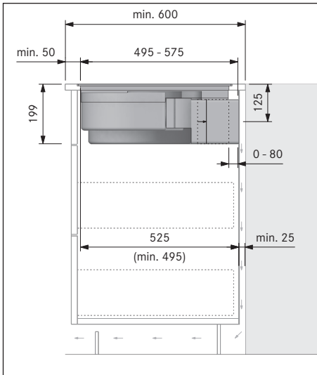
Abb. 10.20 Einbaumaße bei Umluft, Montagevariante A
