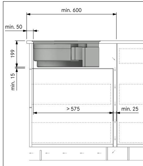
Abb. 10.23 Einbaumaße bei Umluft-Montagevariante B, Arbeitsplattentiefe 600 mm
