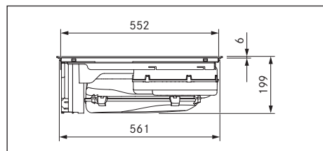
Abb. 3.2 PURSA Gerätemaße Vorderansicht
