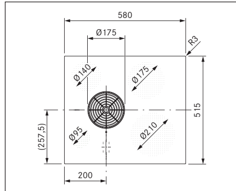
Abb. 3.1 PURSA Gerätemaße Draufsicht
