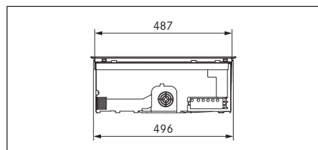
Abb. 3.3 PURSA Gerätemaße Seitenansicht
